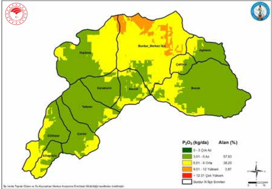
Şekil 2. Burdur İli Topraklarının Fosfor Dağılımları
