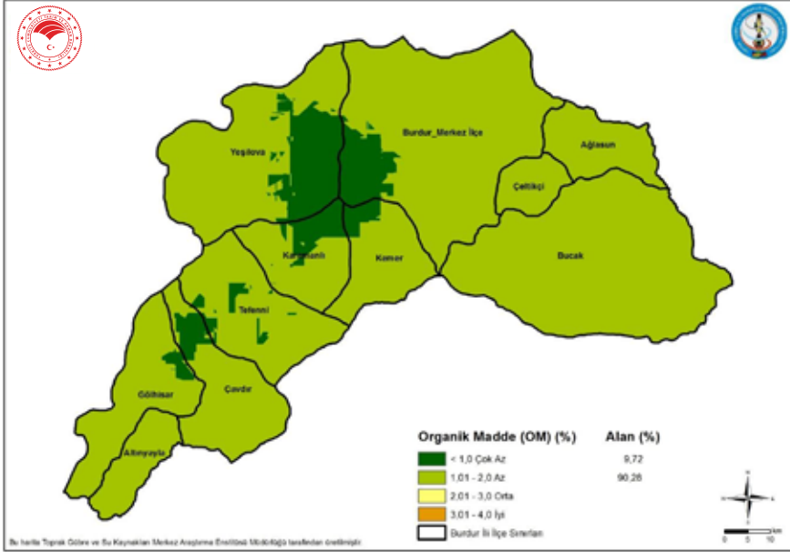
Şekil 1. Burdur İli Topraklarının Organik Madde Dağılımları
