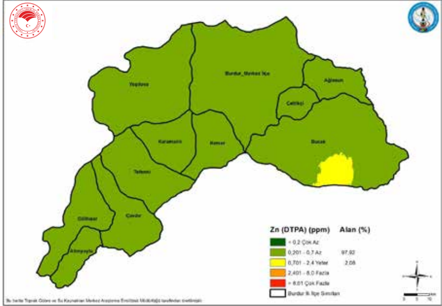
Şekil 6. Burdur İli Topraklarının Çinko Dağılımları
