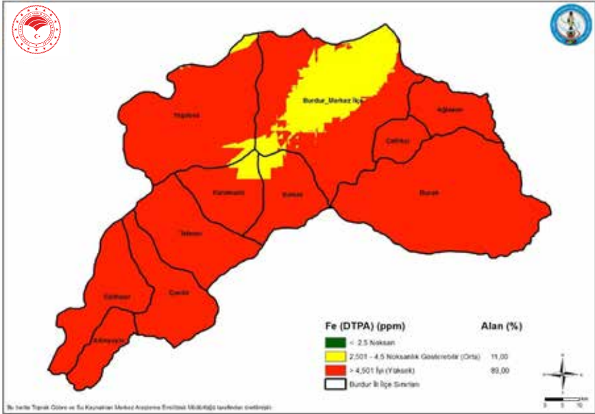
Şekil 4. Burdur İli Topraklarının Demir Dağılımları
