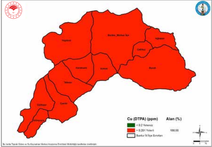
Şekil 5. Burdur İli Topraklarının Bakır Dağılımları
