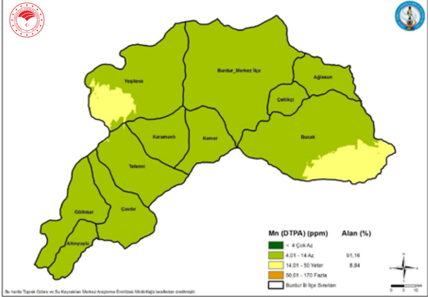
Şekil 7. Burdur İli Topraklarının Mangan Dağılımları
