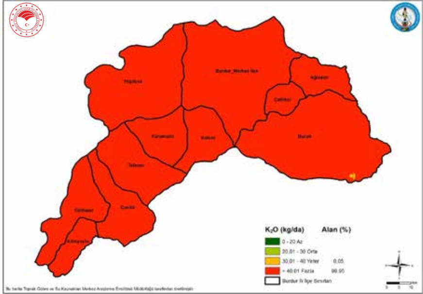
Şekil 3. Burdur İli Topraklarının Potasyum Dağılımları
